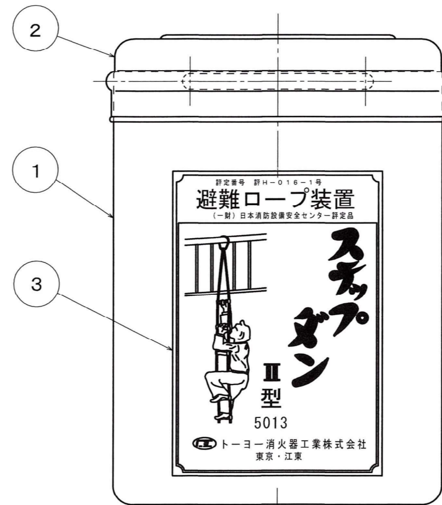
B 矢視図 (正面)
